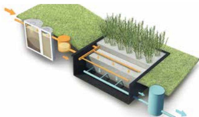
Skica delovanja rastlinske čistilne naprave Limnowet ( www.limnowet.si )
